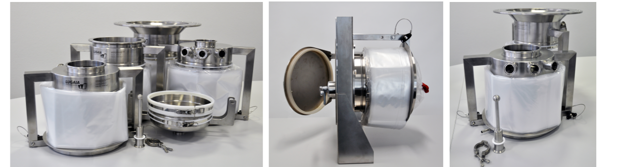
Verschiedene Linerträger mit integriertem Waschsysteem
